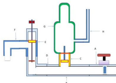
Gambar 3.6 Panjang Bagian Pompa Tektonik
