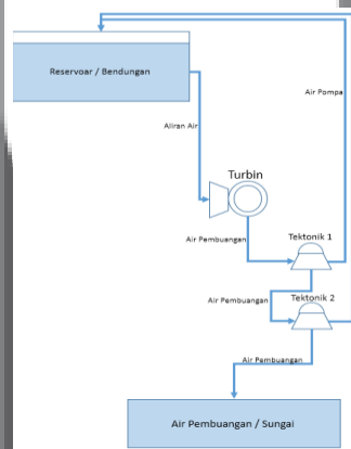
Gambar II-2. Diagram Alir Pompa Tektonik Untuk PLTA Feedback System .
