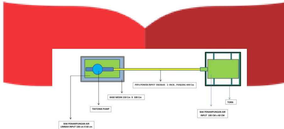
Gambar 3.3 Rancangan Base Pompa
