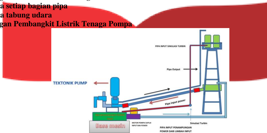
Gambar 3.7 Rancangan Pembangkit Listrik Tenaga Pompa
