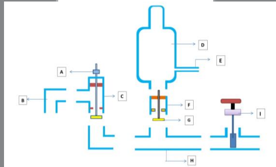
Gambar 3.5 Rancangan Pompa Tektonik
