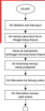
Gambar 4.2 Blok Sistem Kerja Pompa Tektonik
