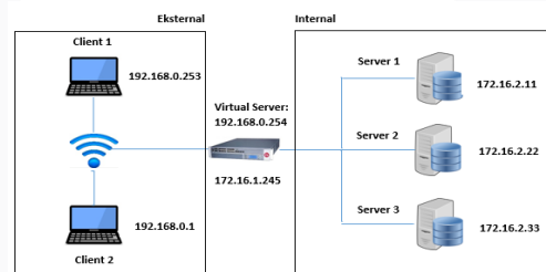
Gambar 3.2 Rancangan Arsitektur
