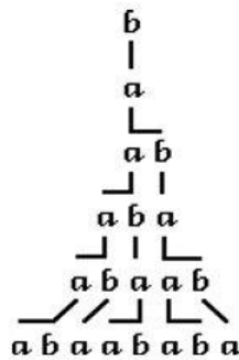
Gambar 2. 4 D0L System Pada Deret Fibonacci[]
