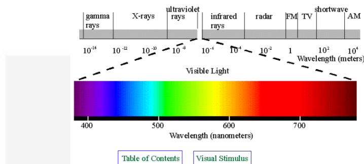
Gambar 2.1 Spektrum cahaya tampak sebagai bagian dari spektrum gelombang elektromagnetik
