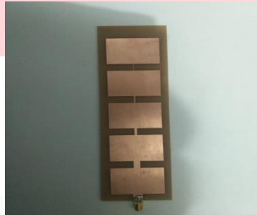
Gambar 3.1 Antena Realisasi
