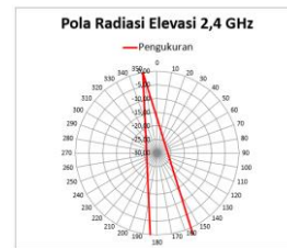
Gambar 3.4 Hasil Pengukuran Pola Radiasi Elevasi
