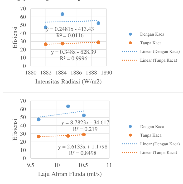
Gambar 7 grafik intensitas radiasi terhadap efisiensi dan laju aliran fluida terhadap efisiensi dengan dan tanpa kaca
