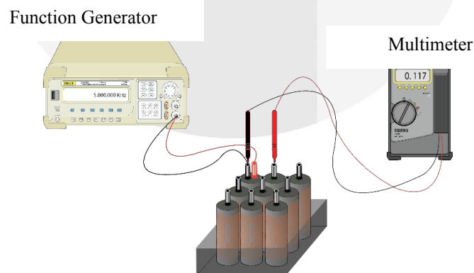
Konfigurasi Koil
