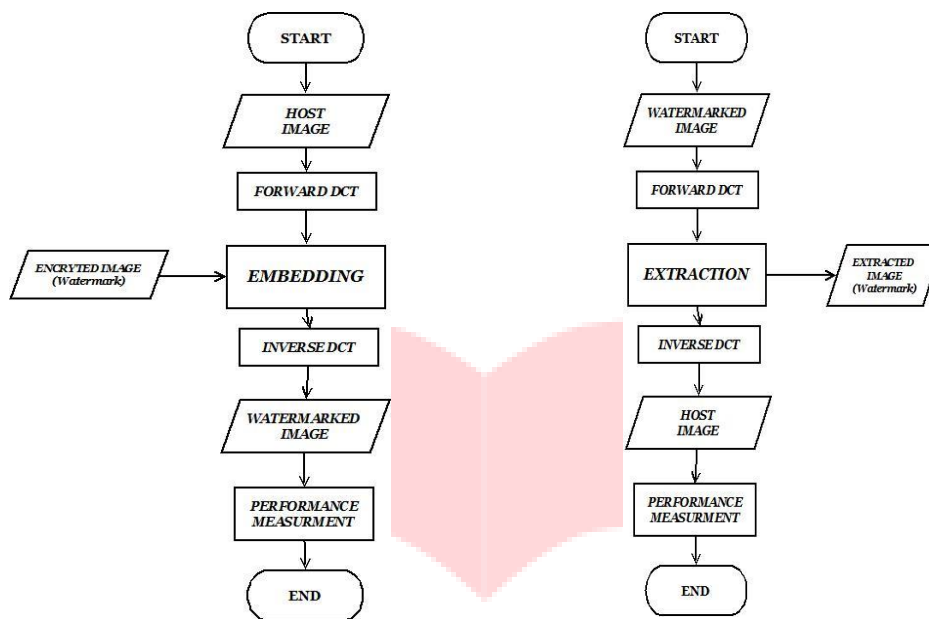
(a) (b) Gambar 2. Diagram Alir Proses (a) Embedding dan (b) Ekstraksi
