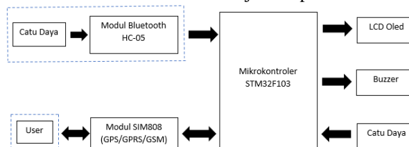
Gambar 2 Diagram Blok Sistem
