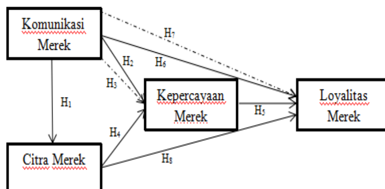
Gambar 2.1 Kerangka Penelitian
