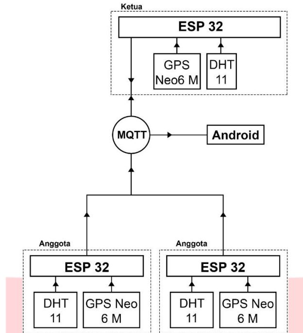
Gambar 2. Blok Diagram.
