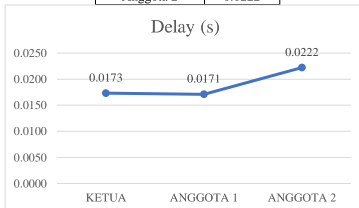
Gambar 4. Grafik Rata-rata Waktu Delay.
