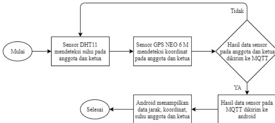
Gambar 3. Diagram Alir Sistem.
