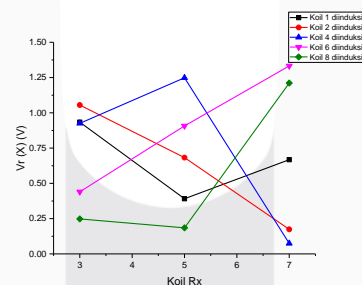
Gambar 3.20 Grafik sampel untuk melihat bentuk objek yang diuji
