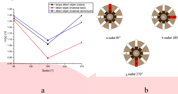
Gambar 3.2 (a) grafik karakteristik koil terhadap sudut, (b) gambar peletakkan sudut antara koil
