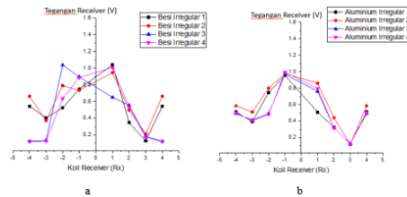
Gambar 3.19 (a) Grafik pada objek Irregular dengan material besi, (b) Grafik pada objek Irregular dengan material aluminium
