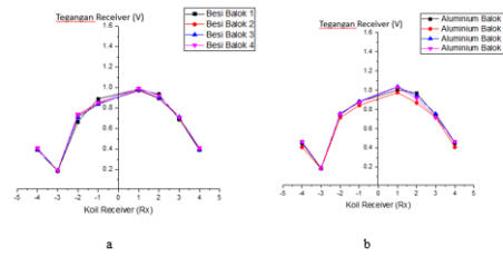
Gambar 3.9 (a) Grafik balok pada koil 1 diinduksi dengan material besi, (b) Grafik balok pada koil 1 diinduksi dengan material aluminium
