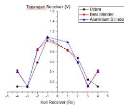
Gambar 3.17 Gambar Grafik koil 7 diinduksi dengan variasi objek udara dan silinder
