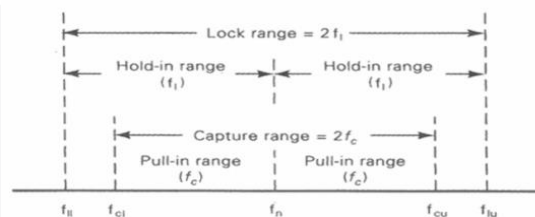
Gambar 2. Gambar Daerah Lock Range dan Capture range [4].
