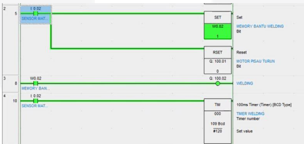
Gambar 11 Simulasi sensor mendeteksi keberadaan raw material
