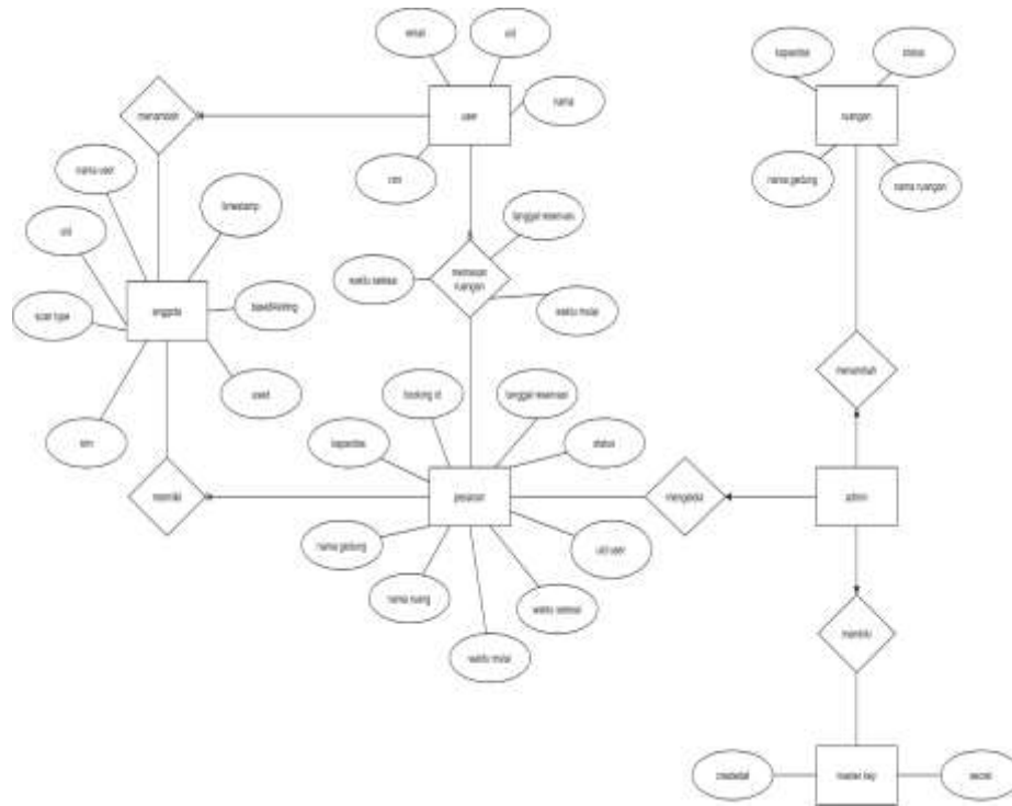
Gambar 3.4 ERD Aplikasi
