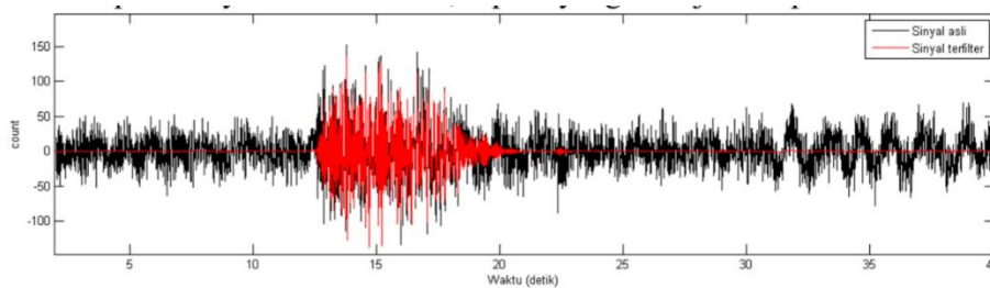
Gambar 2.3 Noise pada sinyal seismik
