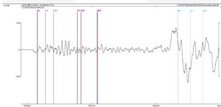
Gambar 2.2 Gelombang P dan Gelombang S
