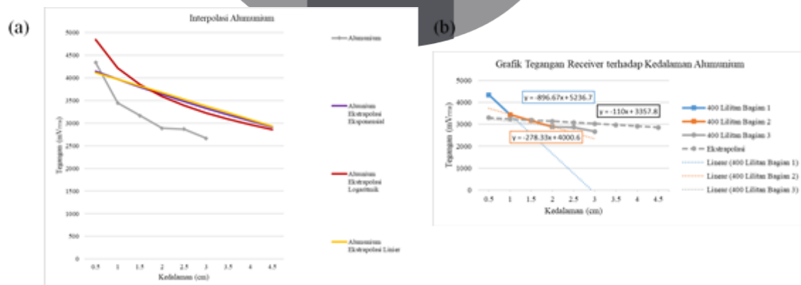
Gambar 9 Hasil ekstrapolasi pada Alumunium (a) Interpolasi Logaritmik, Ekspensial, dan Linier (b) Interpolasi Partisi Linier
