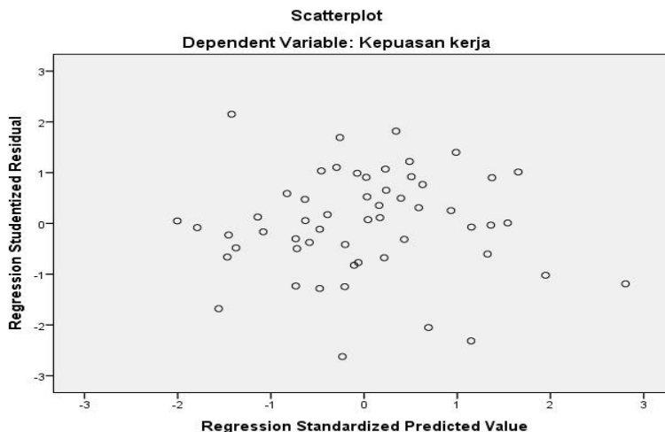
Gambar 1 Grafik Scatterplot Uji Heteroskedastisitas
