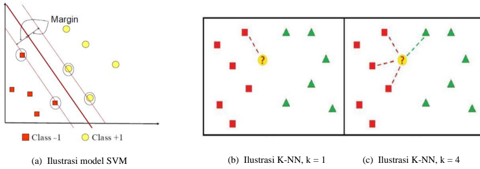
Gambar 2. Ilustrasi klasifikasi SVM (a) [13] dan K-NN (b), (c) [14]
