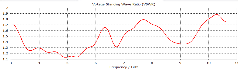
Gambar 5 VSWR.
