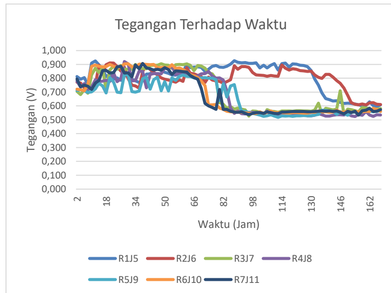
(a) Grafik Pengukuran Tegangan
