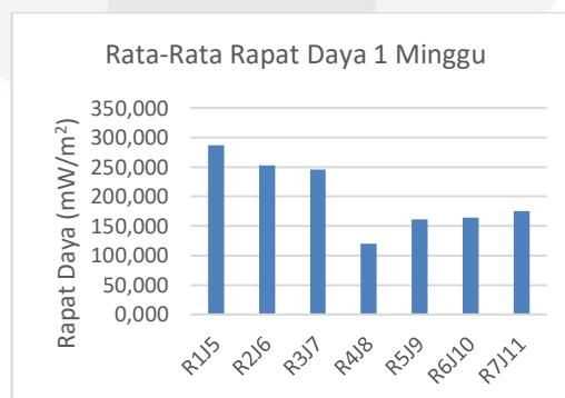
(d) Perbandingan Nilai Rapat Daya Rata-Rata Pada Setiap reaktor
