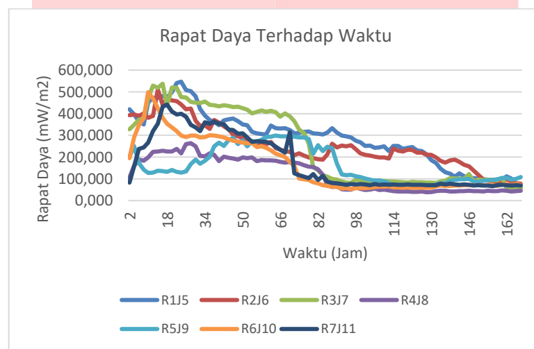
(c) Hasil Perhitungan Rapat Daya selama 7 Hari
