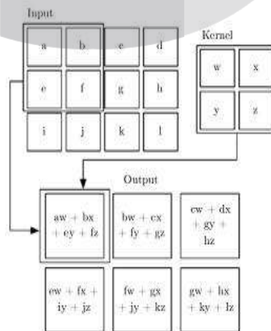
3. Gambar 2. 2 Proses konvolusi pada input array 2D dengan bobot 2D [9]
