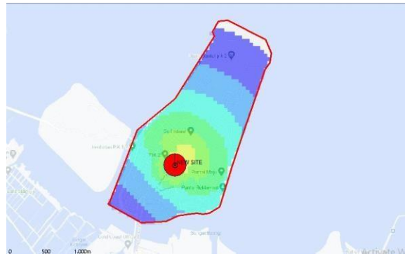
Gambar 4 Penyebaran sinyal RSRP.
