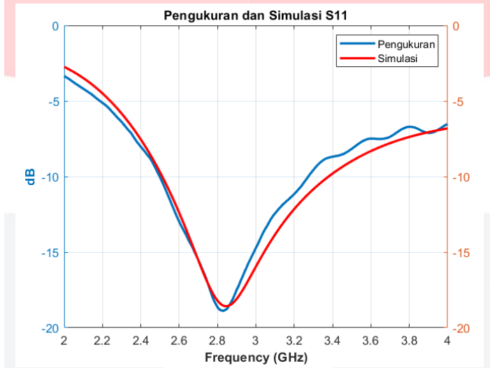
Gambar 4.1 Grafik perbedaan simulasi dan pengukuran return loss port S_{11}
