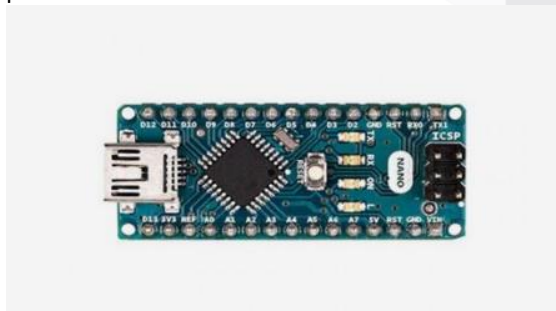
gambar Error! No text of specified style in document. -1 Arduino Nano berikut spesifikasi pada Arduino nano pada tabel dibawah ini
