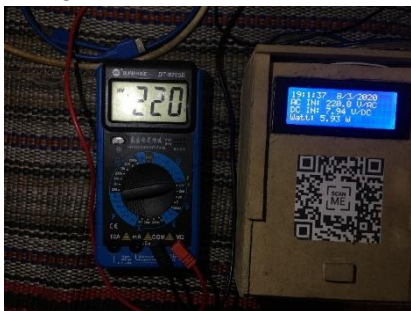
Gambar Error! No text of specified style in document..15 Kalibrasi sensor tegangan ZMPT101B dengan Multimeter
