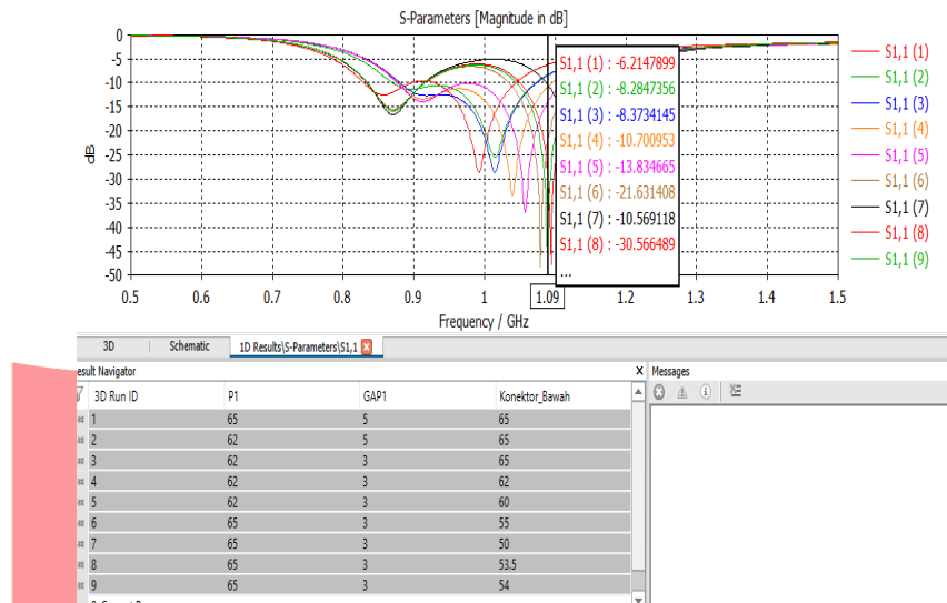
Gambar 3.12 optimalisasi Return Loss penambahan panjang, jarak antar lengan, dan konektor bawah
