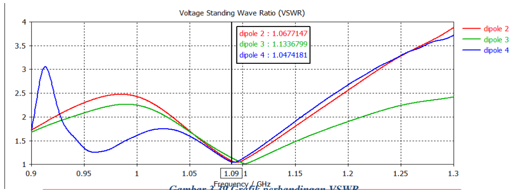
Gambar 3.39 Grafik perbandingan VSWR
