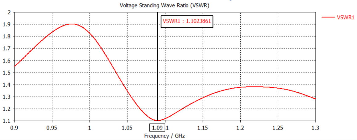
Gambar 3.34 Hasil simulasi VSWR dipole 4
