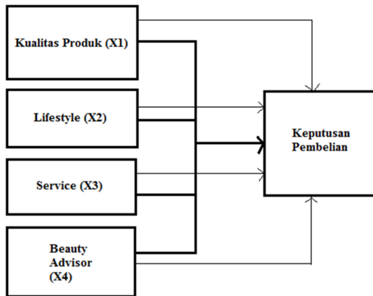
Gambar 2.1 Kerangka Pemikiran
