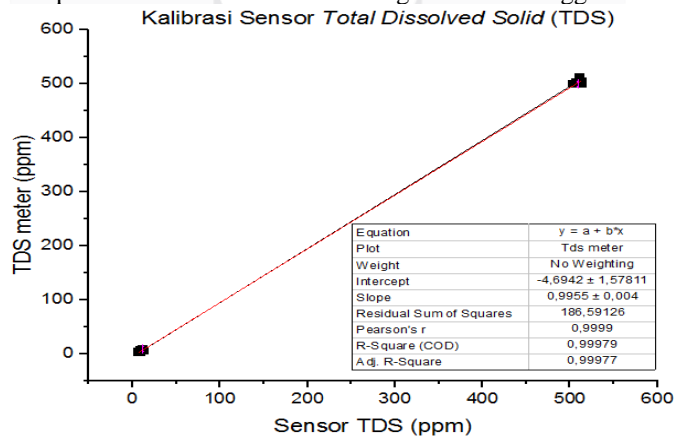
Gambar 7 Grafik Perbandingan Sensor TDS Gravity dengan TDS Meter
