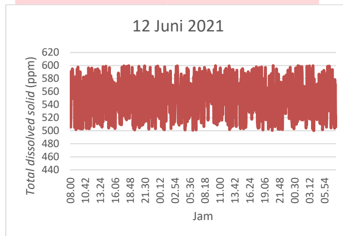
Gambar 13 Grafik Hasil Monitoring TDS Selama Satu Hari
