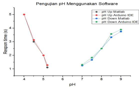
Gambar 10 Grafik Pengujian pH Menggunakan Software
