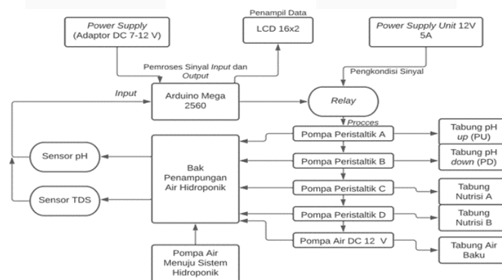
Gambar 1 Desain Sistem Penelitian
