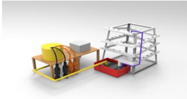
Gambar 2 Desain Sistem Hidroponik
