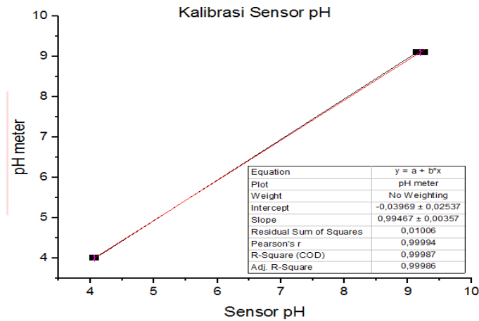
Gambar 6 Grafik Perbandingan Sensor pH dengan pH meter
