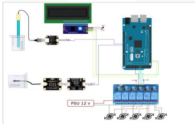
Gambar 4 Wiring perancangan sistem
