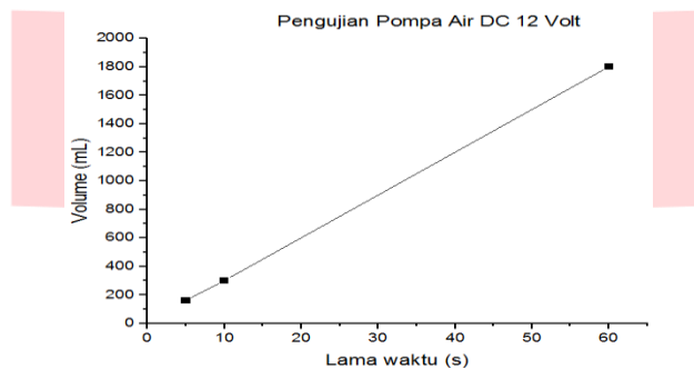
Gambar 8 Grafik Pengujian Aktuator Pompa Air DC 12 12 volt
