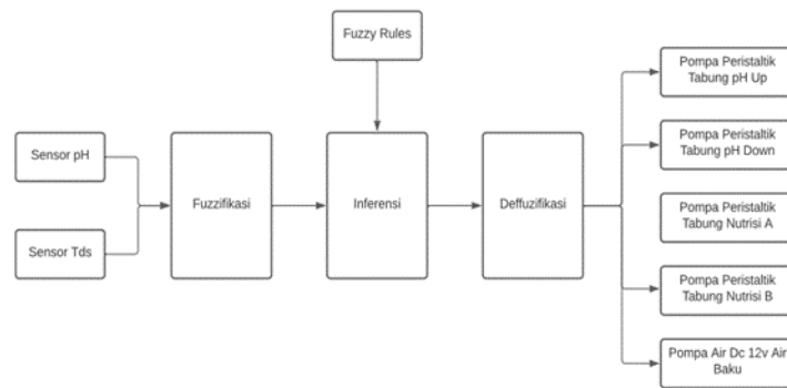
Gambar 3 Perancangan Sistem Fuzzy Logic
