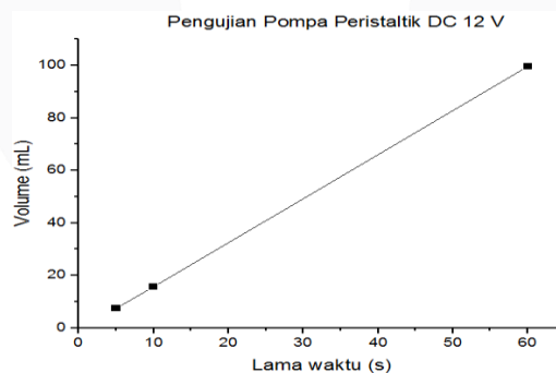
Gambar 9 Grafik Pengujian Aktuator Pompa Peristaltik DC 12 12 volt
