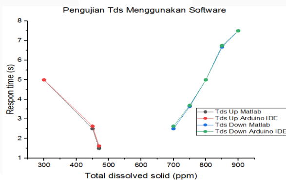
Gambar 11 Grafik Pengujian TDS Menggunakan Software
