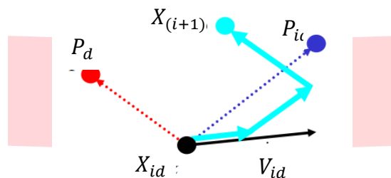
Gambar 1. Ilustrasi dari Algoritma PSO [11]
