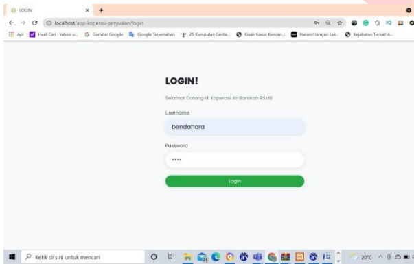
Gambar 4 proses login
