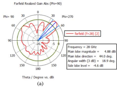
Gambar 10 Simulasi Pola Radiasi Antena
