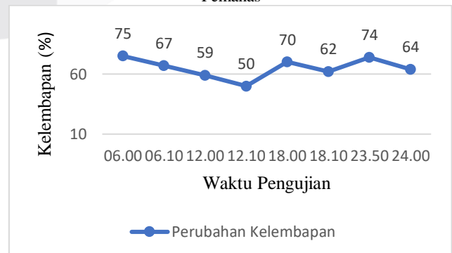
Gambar 7 Grafik Perubahan Kelembapan dengan Pemanas
