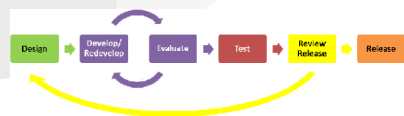
Gambar 1 Metodologi GDLC
