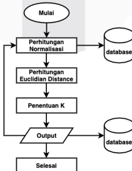
Gambar 4 Tahapan klasifikasi KNN
