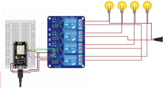
Gambar 3. 5 Rangkaian sistem kendali lampu jarak jauh
