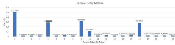
Gambar 11 Grafik Delay Malam Hari (00:42:47 - 00:46:51).
