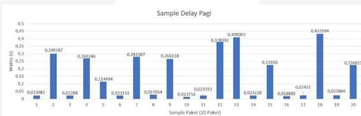
Gambar 8 Grafik Delay Pagi Hari (06:51:26 - 06:56:34).
