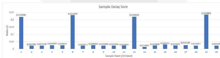
Gambar 10 Grafik Delay Sore Hari (15:24:03 - 15:25:31).
