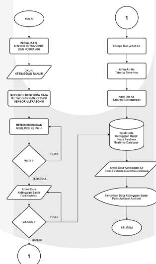
Gambar 2 Diagram Alir Keseluruhan Sistem.
