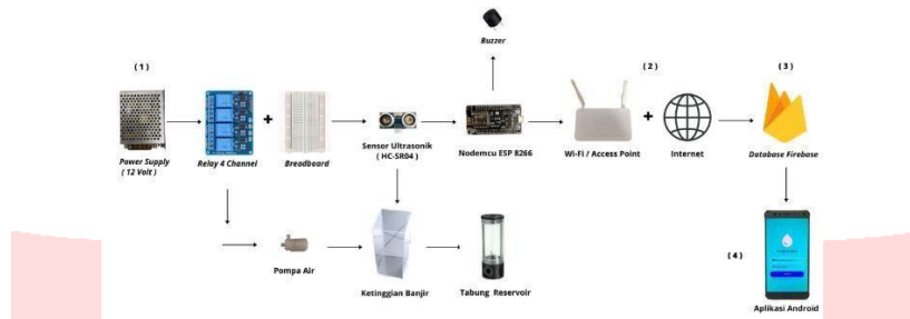
Gambar 1 Desain Sistem.
