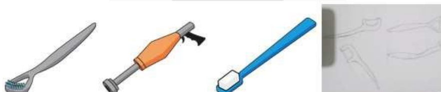
Gambar 3 Item
