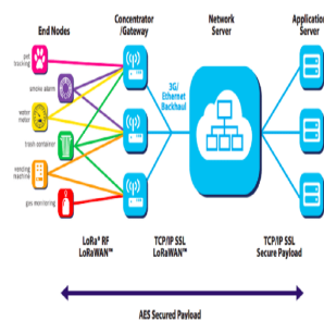
Gambar 1 Arsitektur Jaringan LoRaWAN[5]
