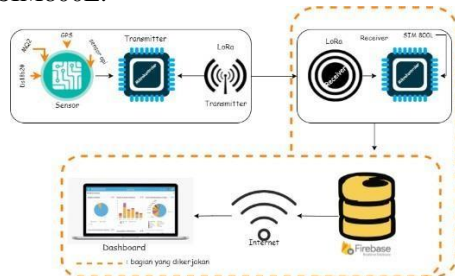
Gambar 2 Desain Sistem
