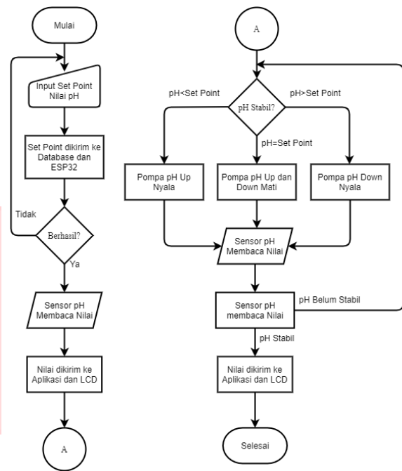
GAMBAR 5 Diagram Alir Sistem
