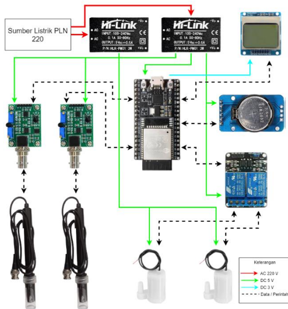
GAMBAR 4 Skematik Rangkaian
