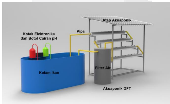
GAMBAR 1 Desain Sistem Akuaponik Secara Keseluruhan
