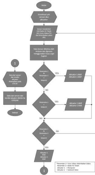
Gambar 3. 8 Desain Alur Perangkat Lunak Pada Arduino Mega
