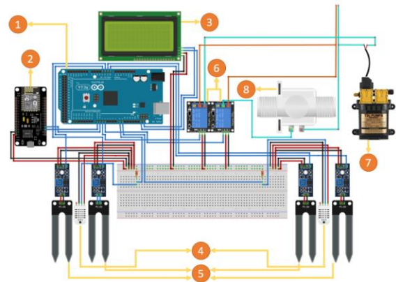
Gambar 3. 1 Desain Perangkat Keras
