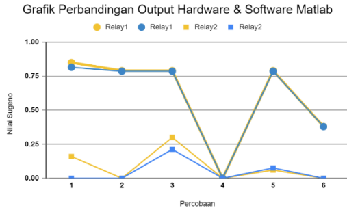
Gambar 4. 3 Grafik Perbandingan Output Hardware dan Software Matlab
