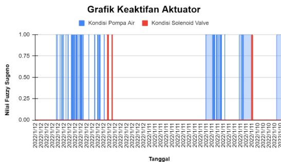
Gambar 4.10 Grafik Keaktifan Aktuator
