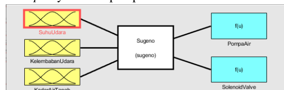
Gambar 3. 4 Variabel Input dan Output
