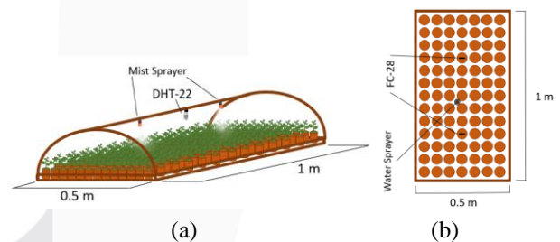
Gambar 3. 2 Desain Sungkup Media Tanam (a) Tampak Samping dan (b) Tampak Atas
