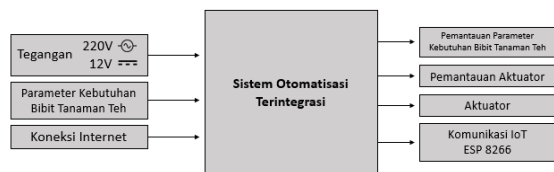
Gambar 3. 1 Desain Konsep Sederhana
