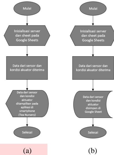
Gambar 3. 3 Desain Alur Perangkat Lunak Pada (a) Tea Monitoring System App dan (b) ESP 8266
