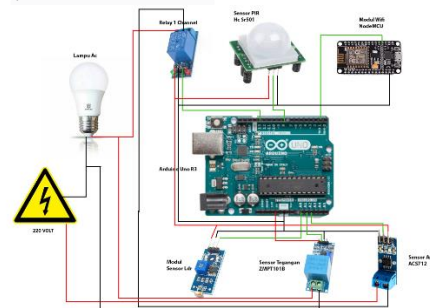
GAMBAR 2. Rangkaian Sistem
