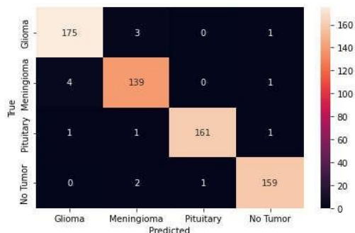
GAMBAR 13 Confusion matrix skenario pengujian terbaik
