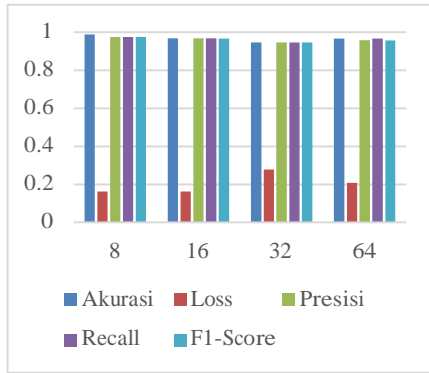
GAMBAR 10 Hasil pengujian skenario batch size
