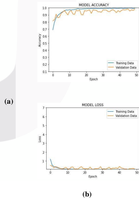
GAMBAR 12 (a) Akurasi dan (b) loss sistem
