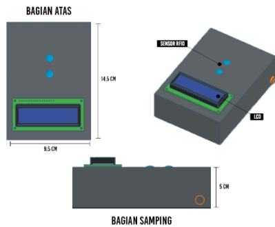
GAMBAR 3.5. Rancangan Box Perangkat Keras.
