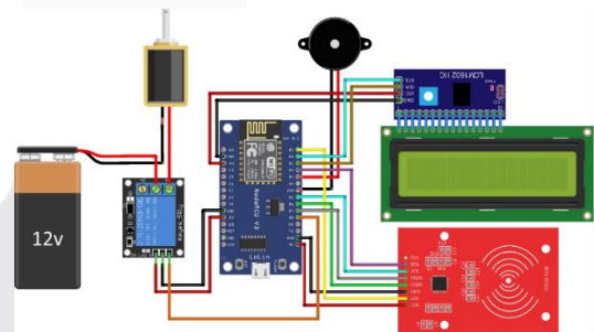
GAMBAR 3.4. Rangkaian Schematic Perangkat Keras.
