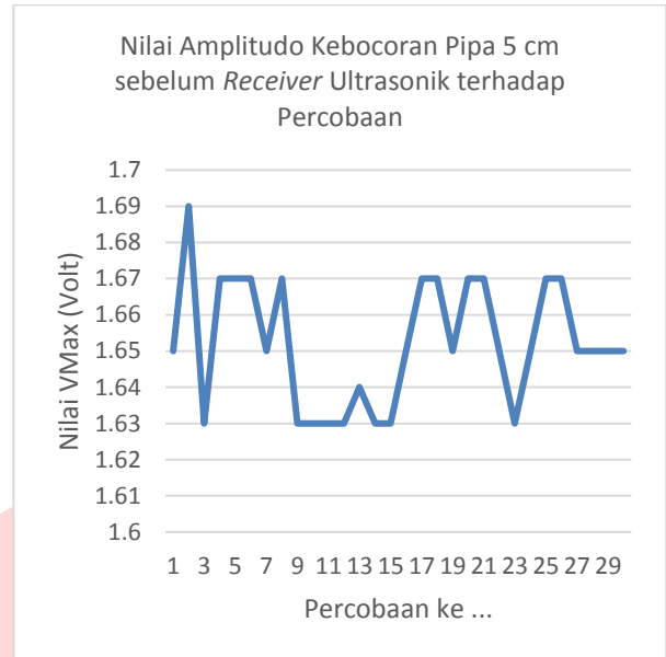
GAMBAR 10 Data nilai Amplitudo kondisi Pipa Bocor 5 cm dari Receiver Ultrasonik
