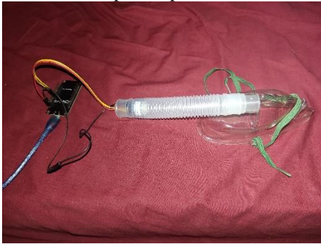
Gambar 1 Desain Perangkat Keras
