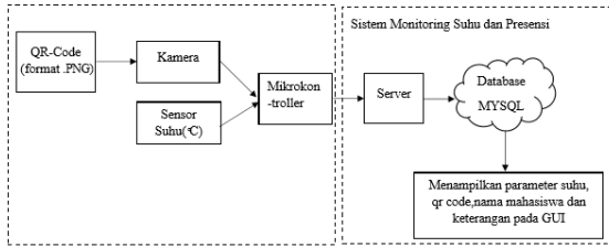
GAMBAR III.1 Diagram Keseluruhan Sistem
