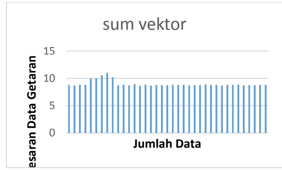
GAMBAR 4.4 Grafik MPU6050 Dalam Kondisi Getaran Kipas Dengan Beban Isolasi
