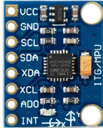
GAMBAR 3.4 MPU 6050
