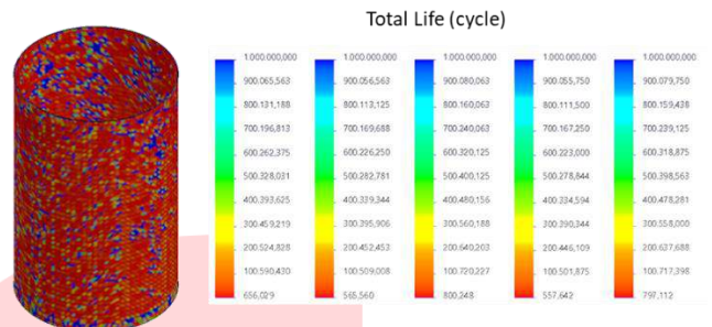
GAMBAR. 6 Hasil simulasi kelelahan pada ponton drum yang sebenarnya
