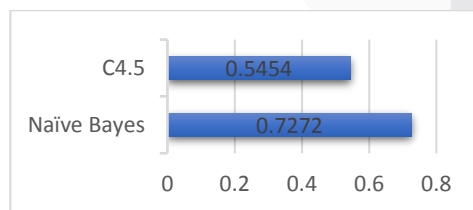
GAMBAR 3. PERBANDINGAN AKURASI
