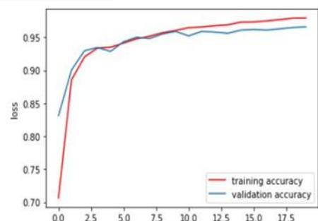
GAMBAR 11 GRAFIK AKURASI RASIO 90:10
